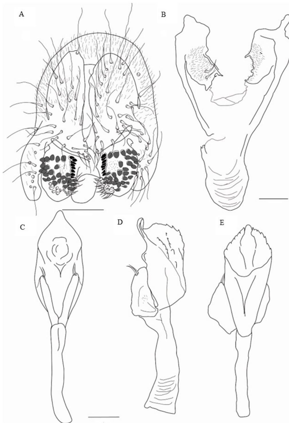
Figura 8. Drosophila ulba sp. nov. Genitalia ♂ A , epandrio, cerco, surestilo. B , hipandrio y gonopodios en vista ventral. C , D , E , edeago y paráfisis en vista ventral, lateral y dorsal, respectivamente. Escalas: 100 \mu m.
