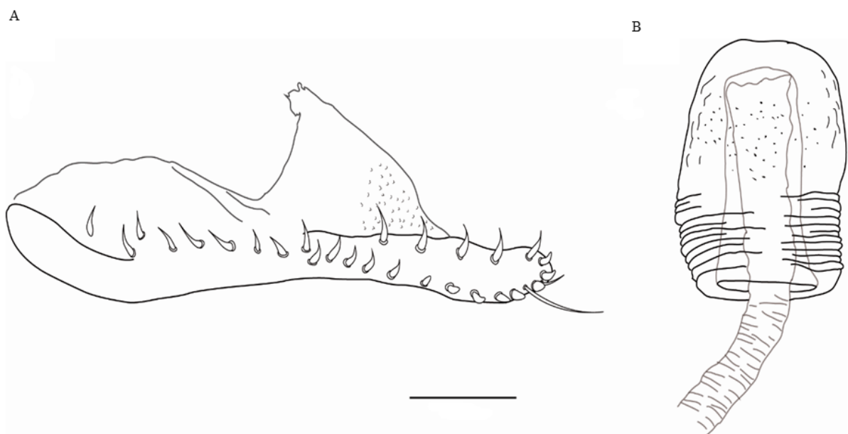
Figura 9. Drosophila ulba sp. nov. Genitalia ♀ A , oviposito, vista lateral. B , espermateca. Escala: 100 µm.
